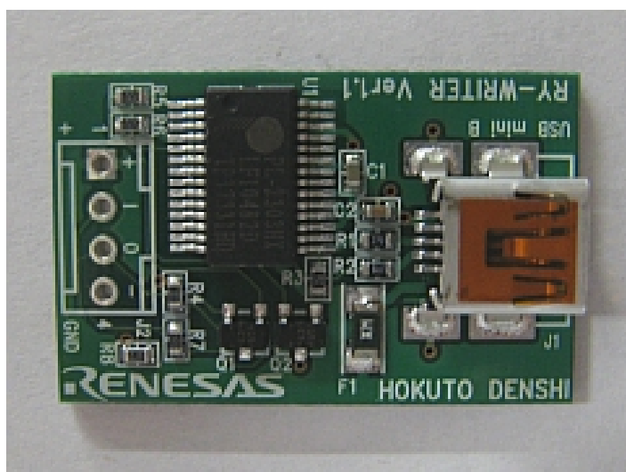
RY-WRITER基板
