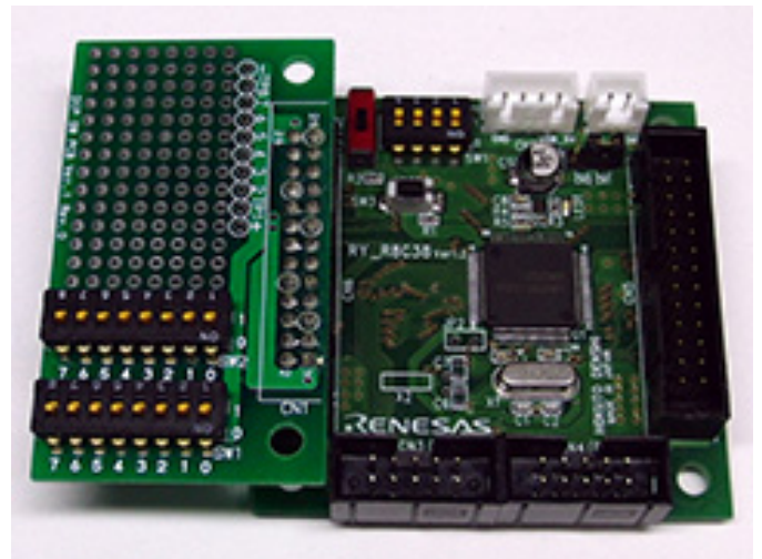
部品を実装し、RY_R8C38ボードに取り付けた例 ※R8C38ボード DIPスイッチ基板以外は、別売です。
