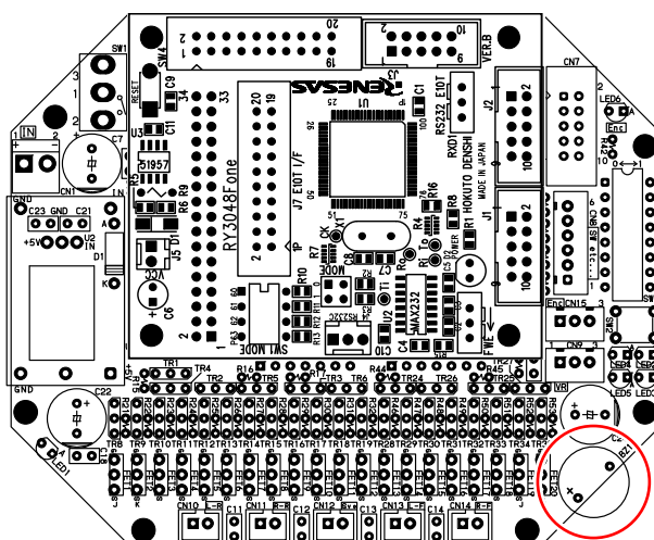
モータドライブ基板 TypeS Ver.2
