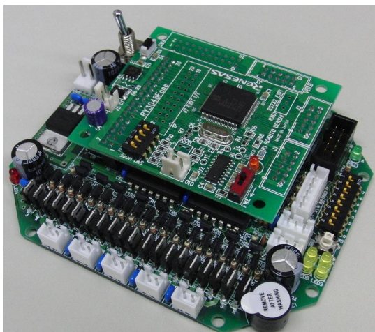
▲モータドライブ基板 TypeS Ver.2
